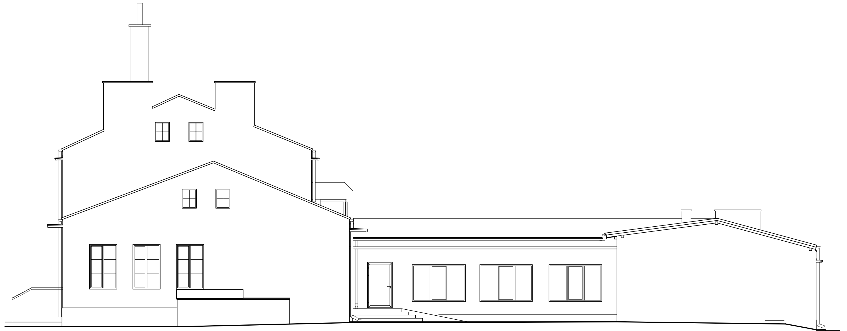
ELEWACJA ZACHODNIA 1:100
