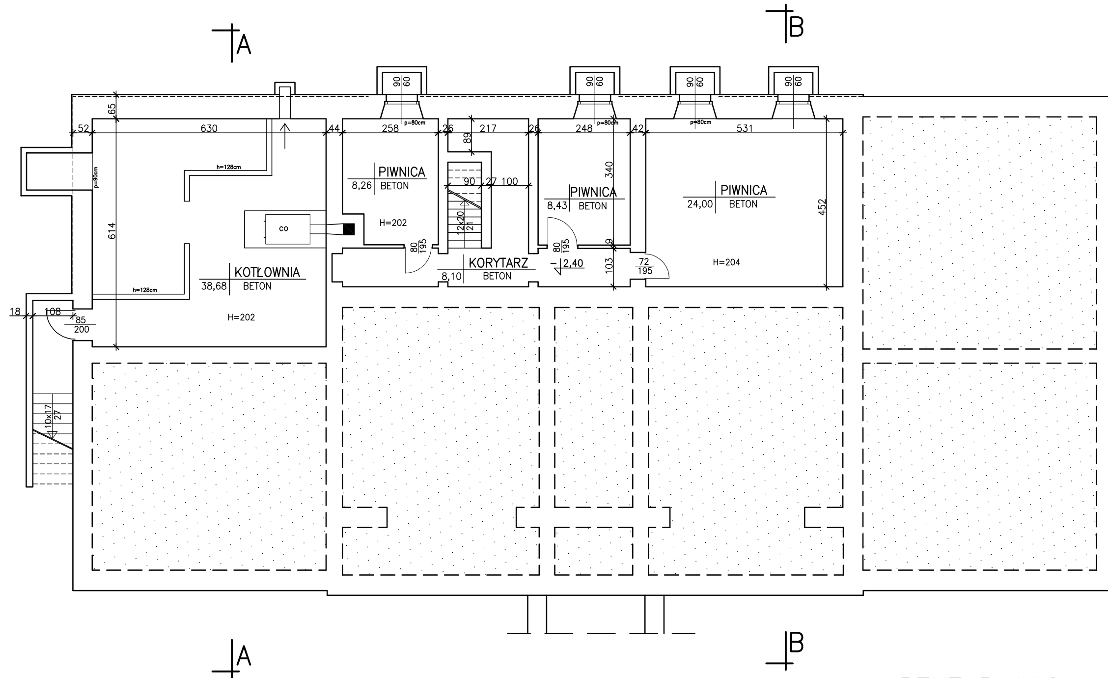
RZUT PIWNIC 1:100
